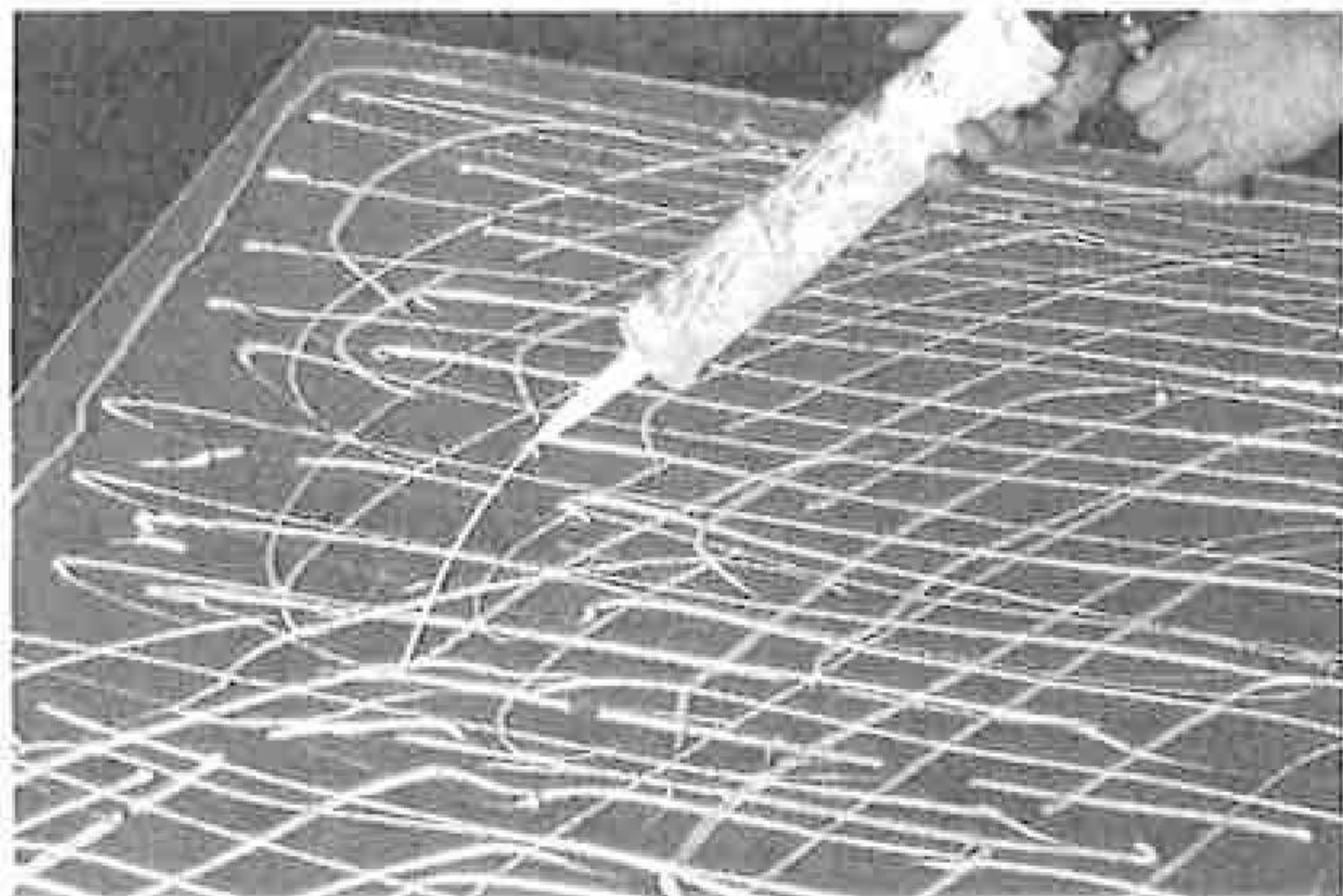
塗布するだけで防音・防振機能を持つ「グリーングロ」
